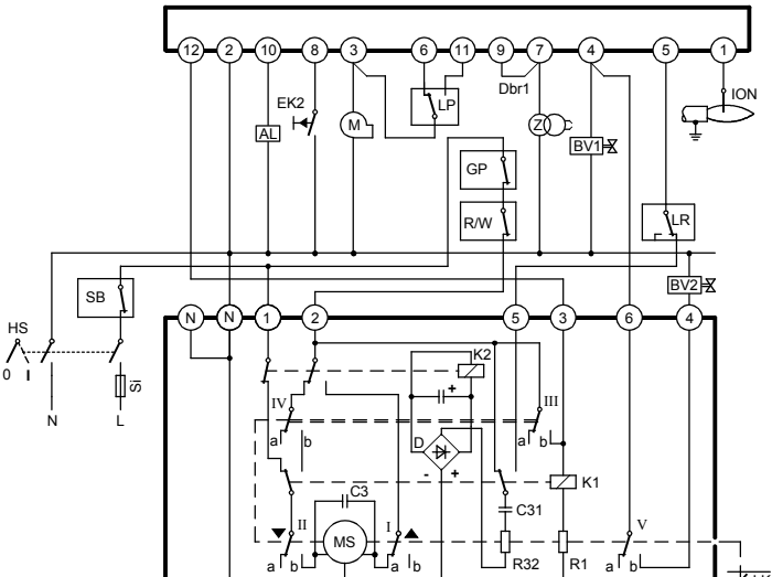
SQN91.140... / 2-х контурное регулирование
