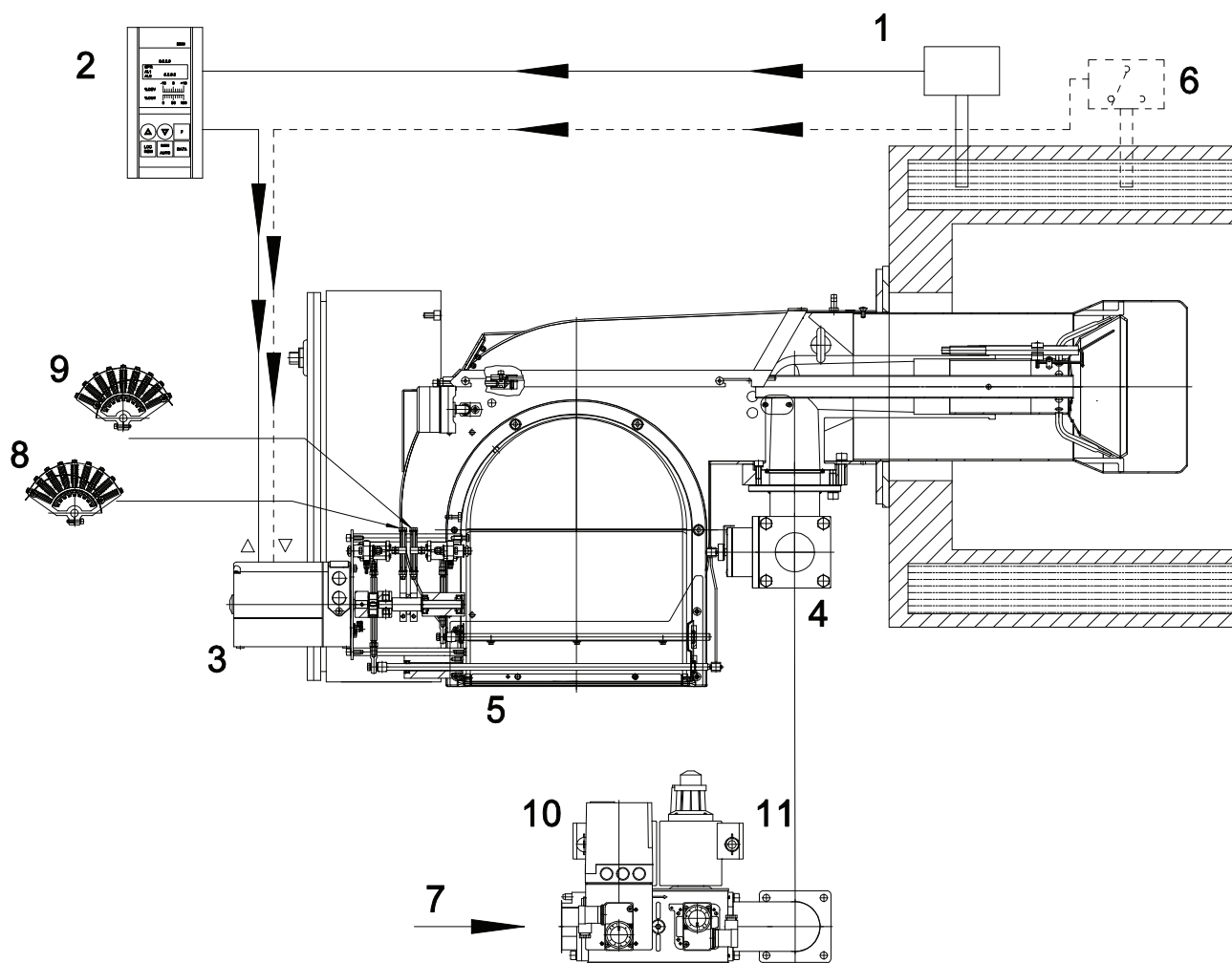
Fig. 13 ПРИНЦИП РАБОТЫ
