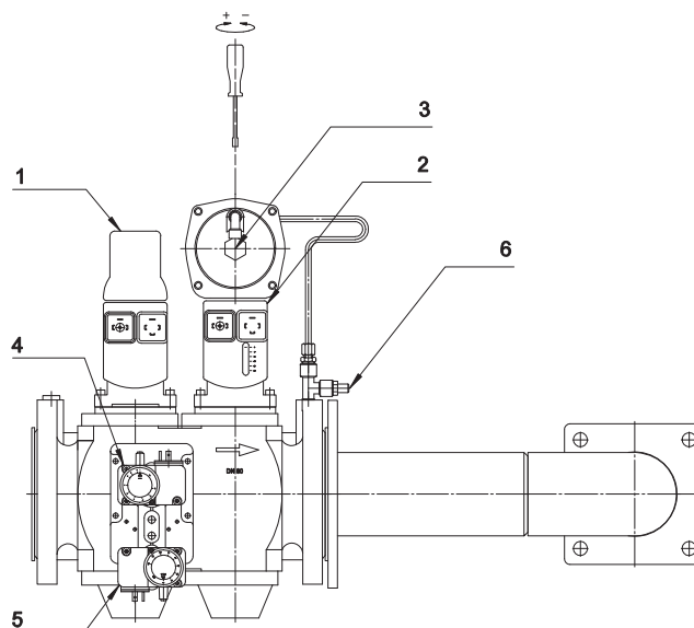
Fig. 19 ОСНОВНАЯ ГАЗОВАЯ РАМПА: SIEMENS VGD40...
