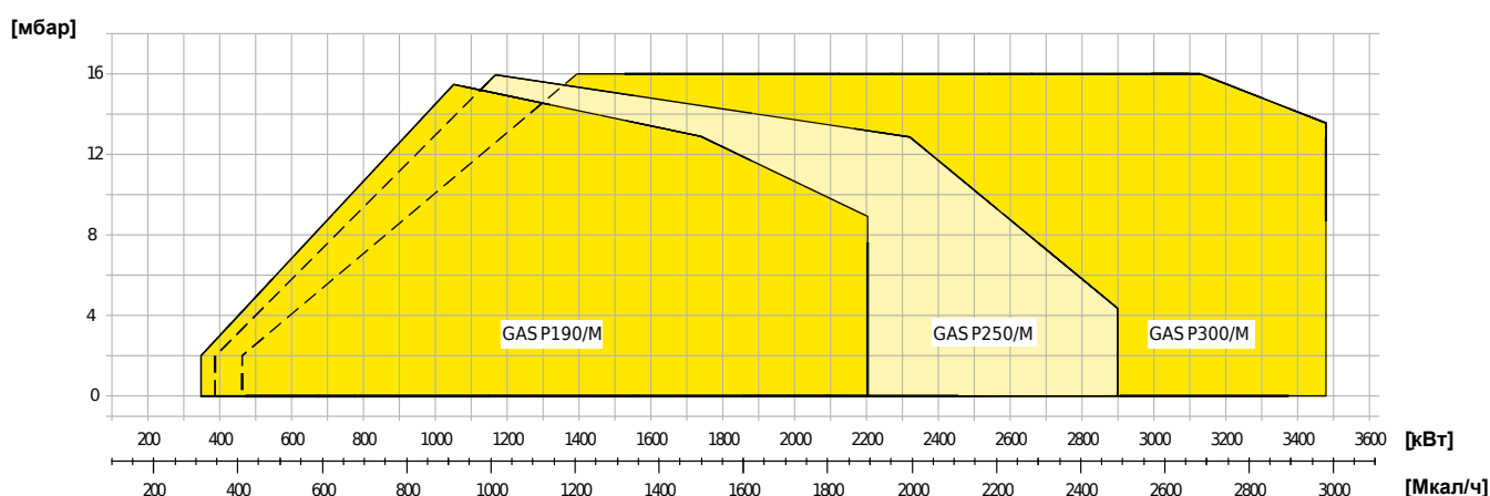
Fig. 1 X = Мощность Y = Сопротивление камеры сгорания
