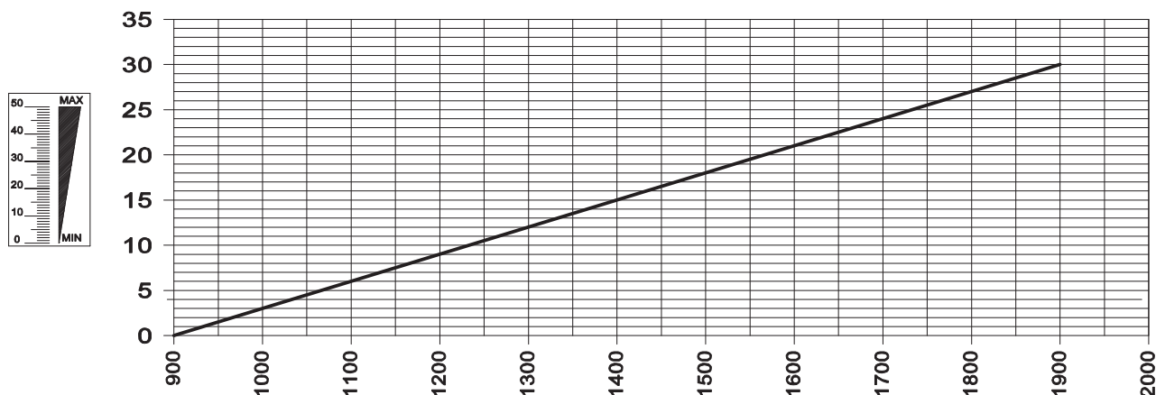
Fig. 30 Ось X= Мощность [Мкал/ч] ; Ось Y= к-во отметок
