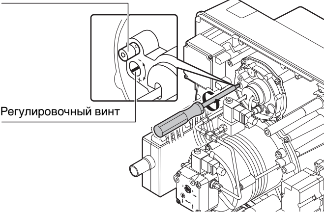
Индикаторный винт
