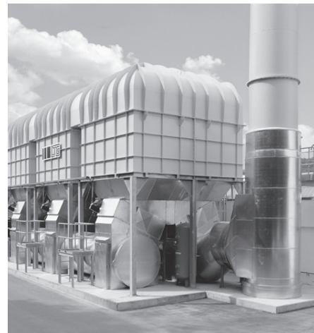
Установка очистки и регенерации газа
