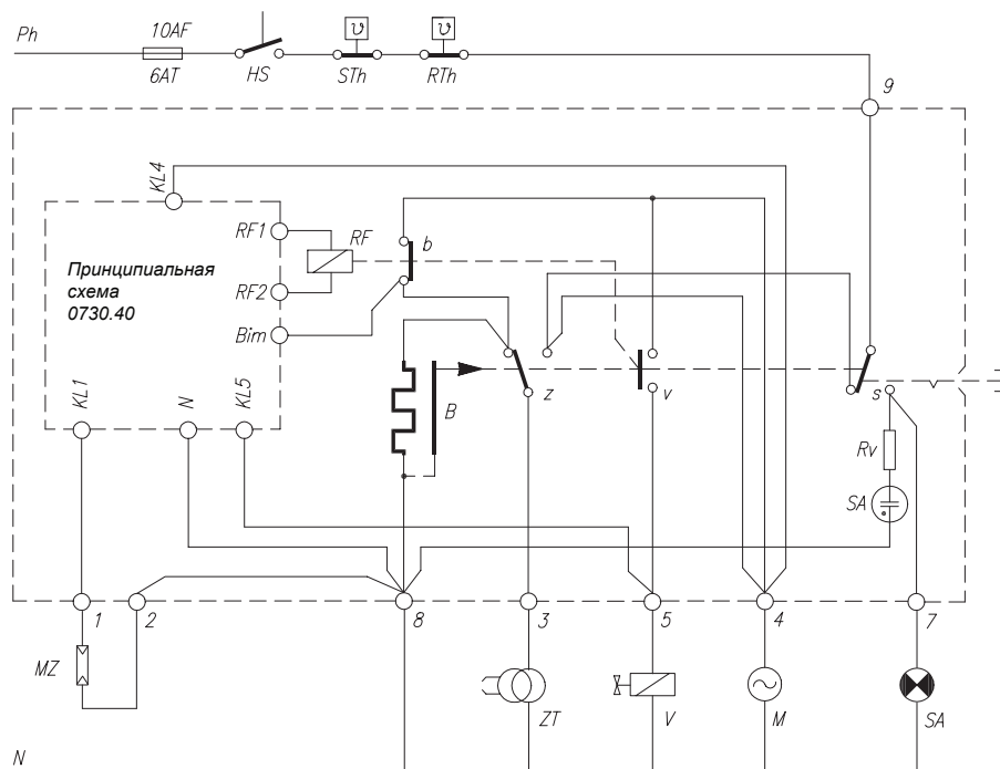
Электросхема TFI 830.3
