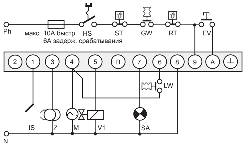
Схема соединений и диаграмма протекания программного цикла для DMG 976
