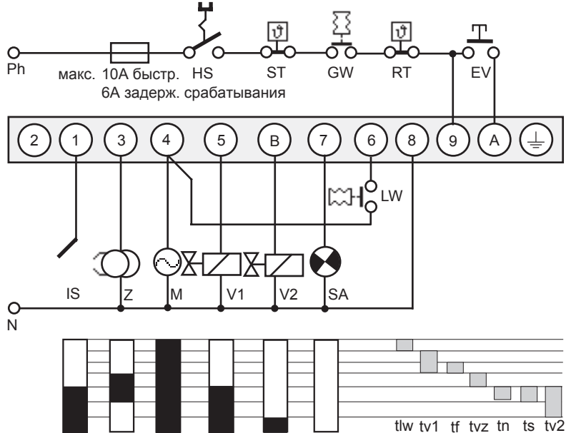
Схема соединений и диаграмма протекания программного цикла для DMG 976
