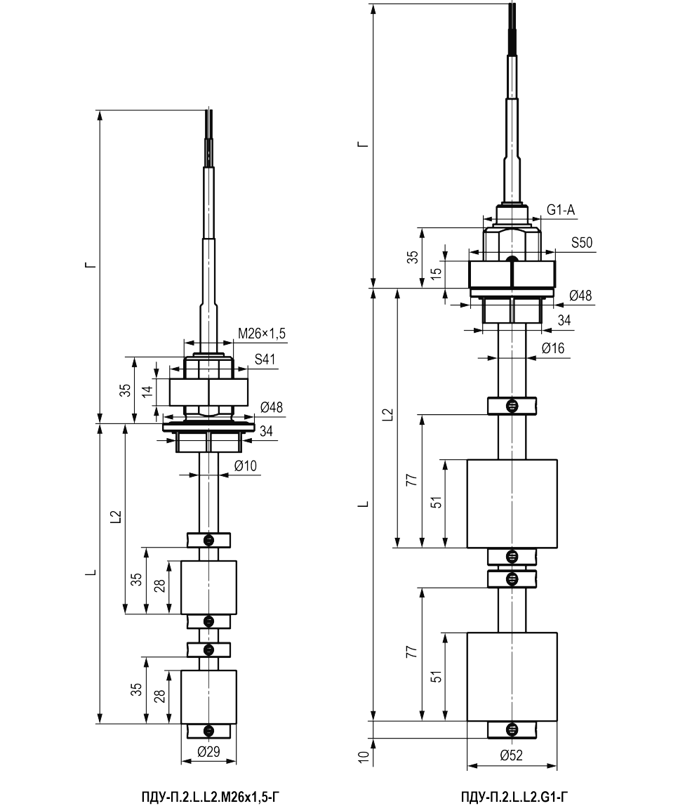
Рисунок 3 – Габаритные и присоединительные размеры двухуровневых ПДУ-П с кабельным выводом
