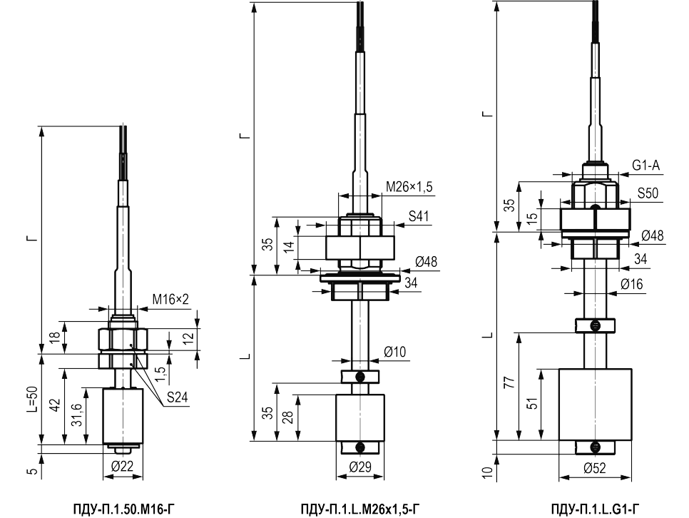
Рисунок 2 – Габаритные и присоединительные размеры одноуровневых ПДУ-П с кабельным выводом
