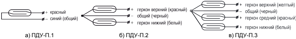
Рисунок 5 – Схемы внутренних соединений проводов
