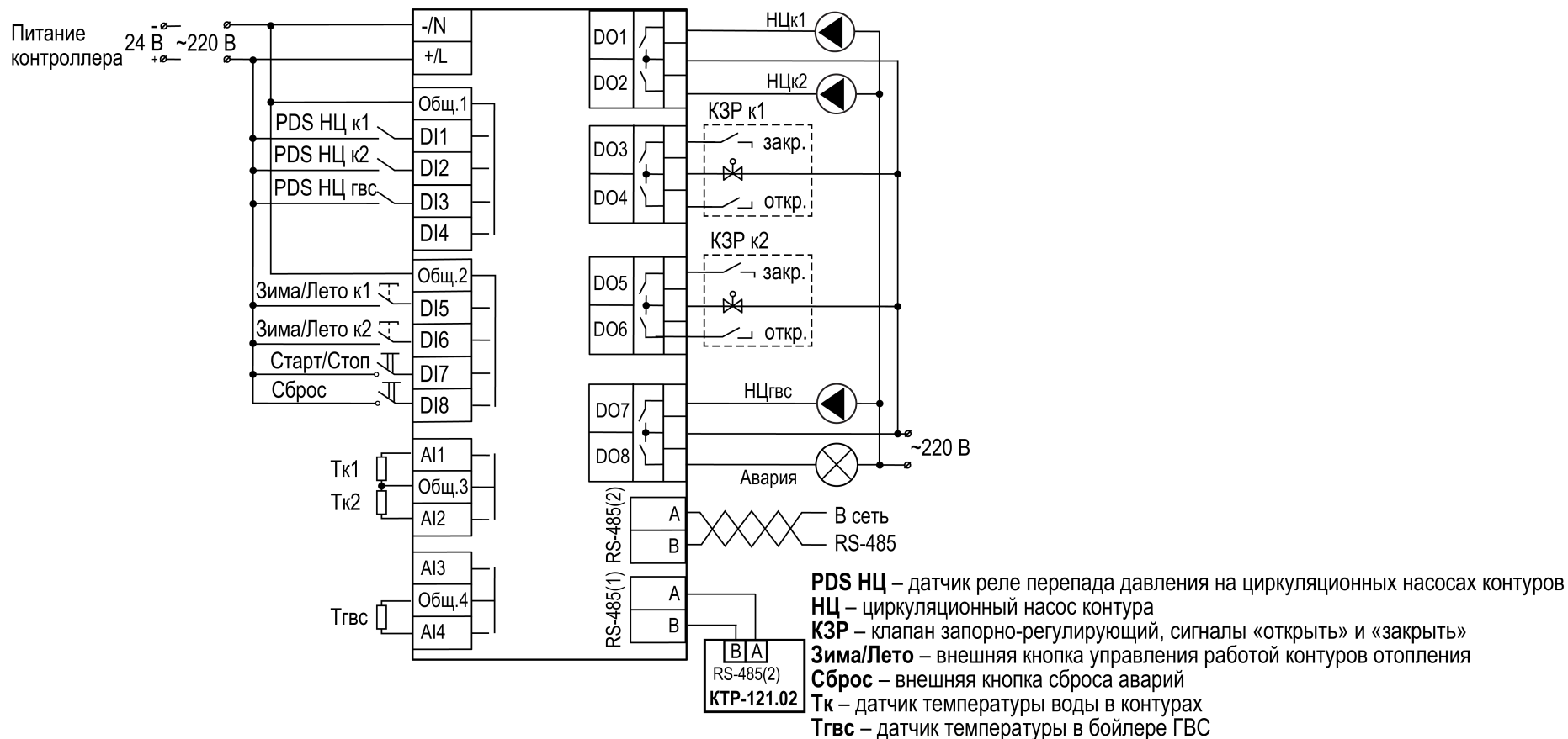
Рисунок 7.4 – Схема подключения KTR-121.03.10 для управления контурами ГВС и отопления
