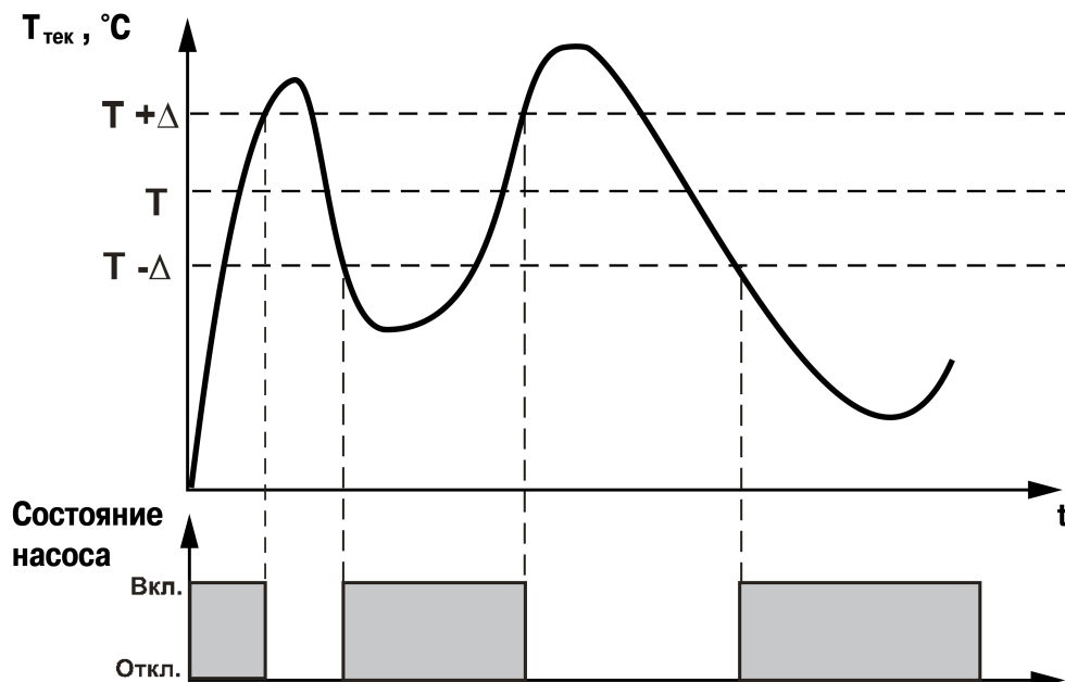
Рисунок 10.2 – Регулирование температуры в зависимости от времени включения насоса
