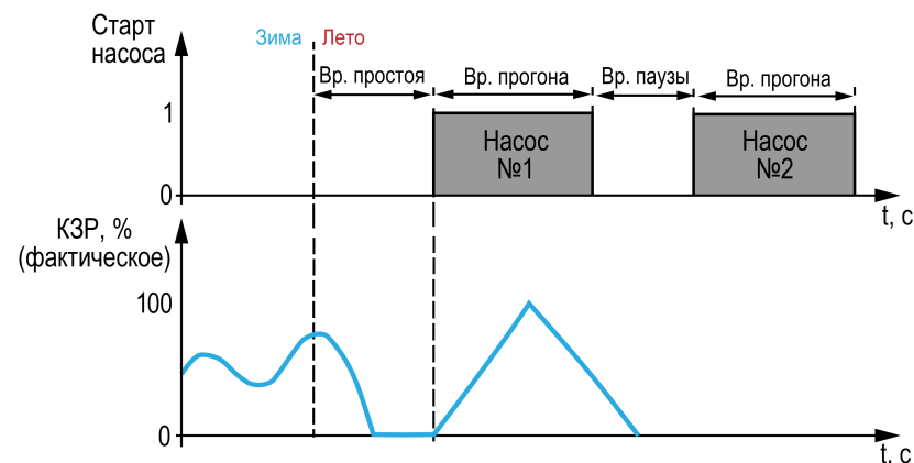
Рисунок 10.10 – Прогон при сезоне «Лето»
