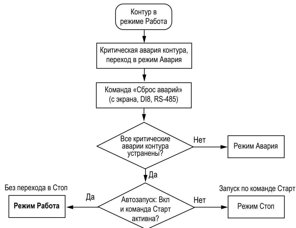
Рисунок 10.11 – Автозапуск контура после критической аварии
