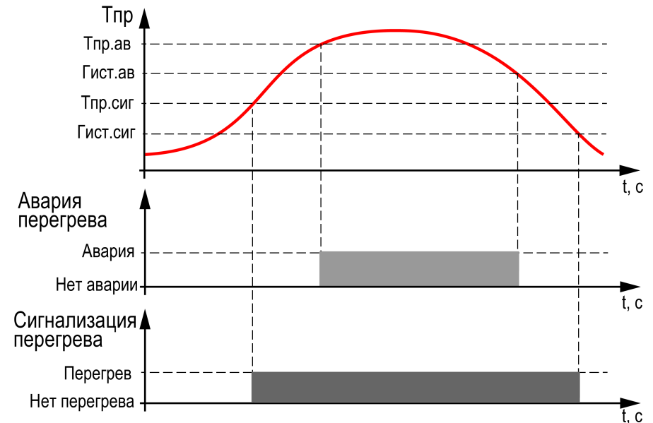
Рисунок 10.12 – Принцип определения и сброса аварии и сигнализации перегрева
