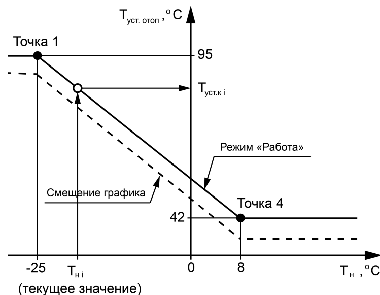
Рисунок 10.8 – Отопительный график
