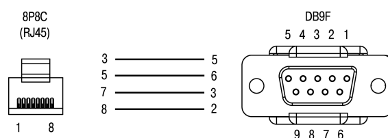
Рисунок 5.21 – Схема кабеля KC16
