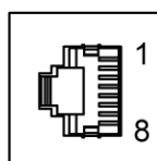
Рисунок 5.23 – Контакты порта Ethernet
