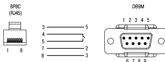
Рисунок 5.22 – Схема кабеля KC17
