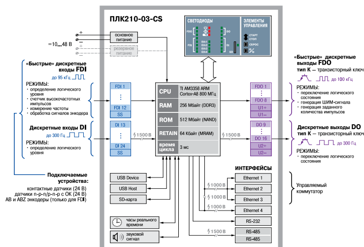
Рисунок 3.3 – Функциональная схема ПЛК210-03-KR
