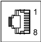
Рисунок 5.19 – Контакты RS-232
