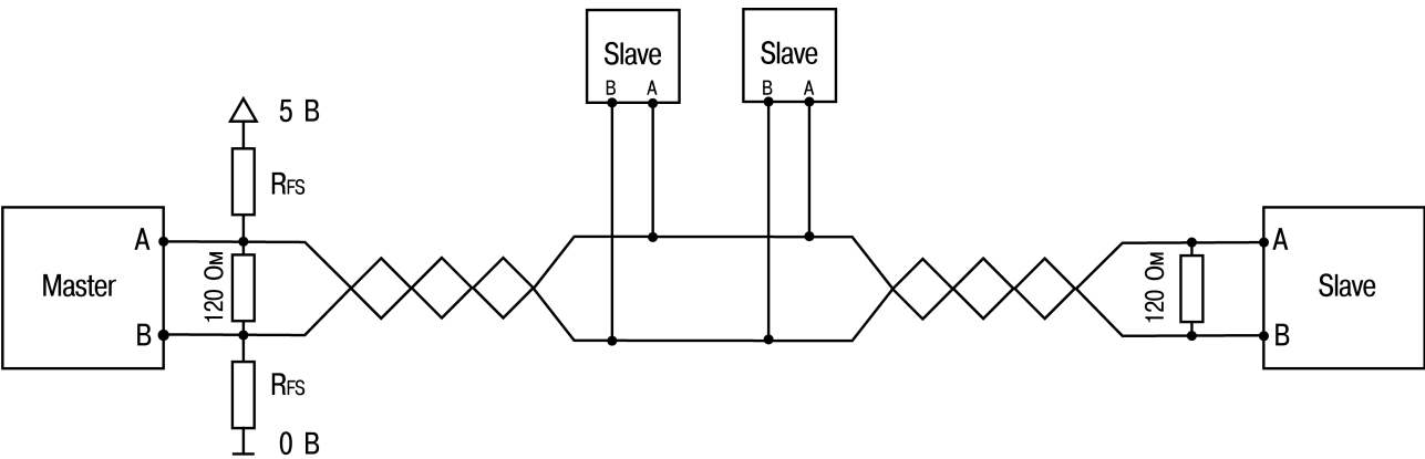
Рисунок 5.18 – Сеть RS-485 с подтягивающими резисторами
