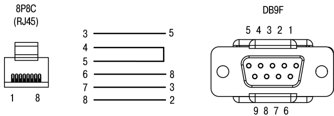
Рисунок 5.20 – Схема кабеля KC14
