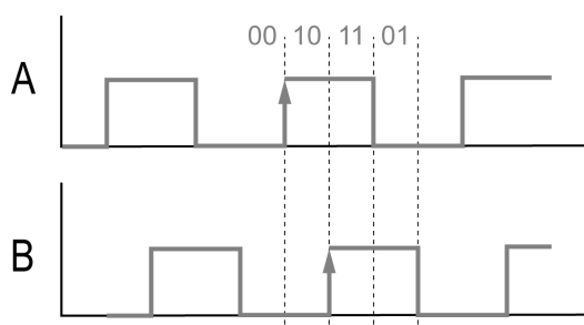
Рисунок 5.11 – Сигналы на выходах инкрементального энкодера при вращении по часовой стрелке
