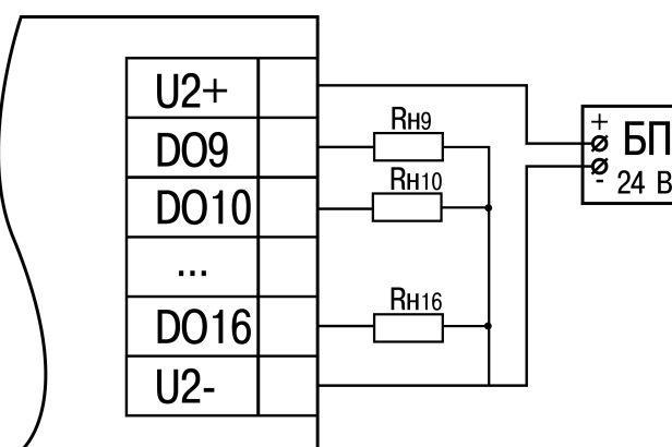
Рисунок 5.14 – Схема подключения внешних связей к дискретным выходам типа «транзисторный ключ» (DO9–DO16)
