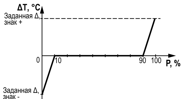
Рисунок 10.11 – Коррекция уставки по тепловой нагрузке потребителя
