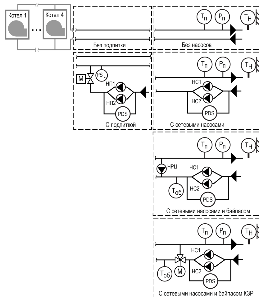
Рисунок 1.1 – Объект управления
