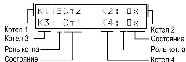
Рисунок 10.12 – Отображение ролей котлов на индикаторе
