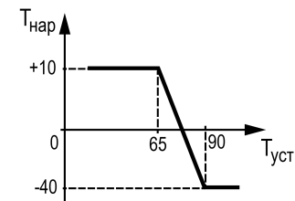
Рисунок 10.10 – График зависимости температуры уставки от наружной температуры
