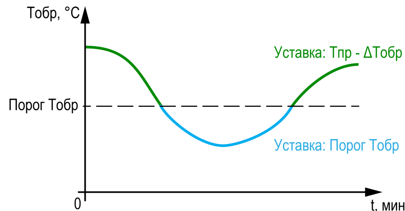
Рисунок 10.11 – Ограничение минимального значения уставки Тобр
