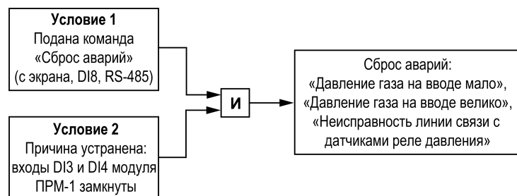
Рисунок 11.1 – Сброс аварий по давлению газа
