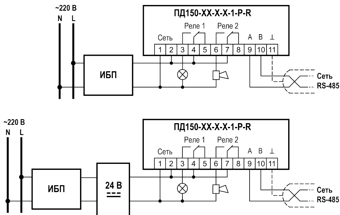
Рисунок 5.5 – Пример схемы подключения преобразователя с интерфейсом RS-485 через ИБП
