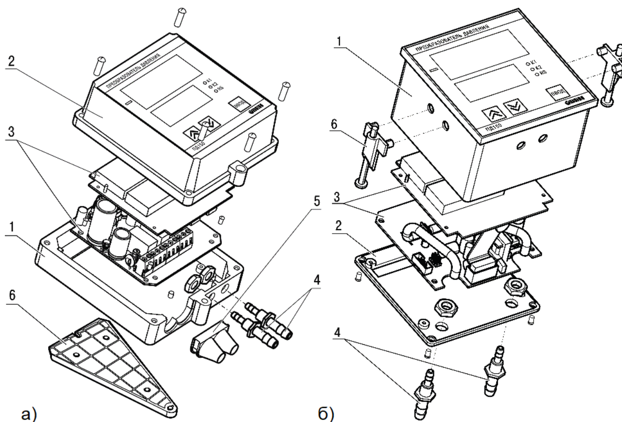
Рисунок 4.1 – Конструкция преобразователя ПД150-ДД настенного (а) и щитового (б) исполнения
