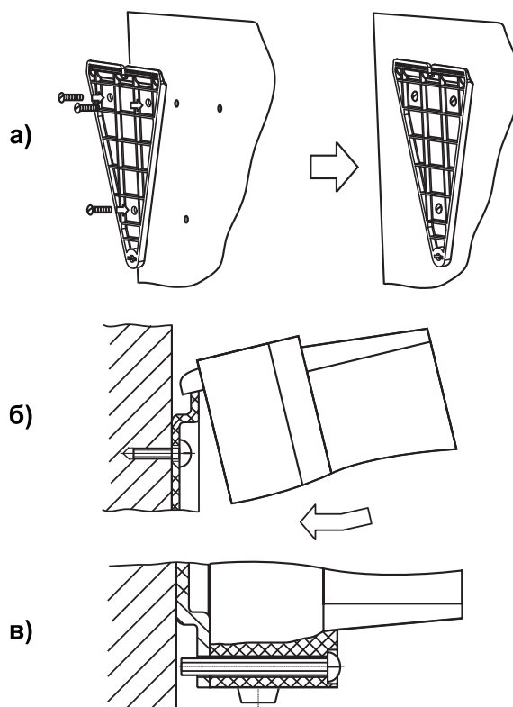
Рисунок 4.2 – Монтаж преобразователя настенного исполнения
