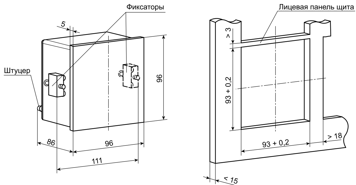
Рисунок 4.5 – Габаритные и установочные размеры преобразователя щитового исполнения
