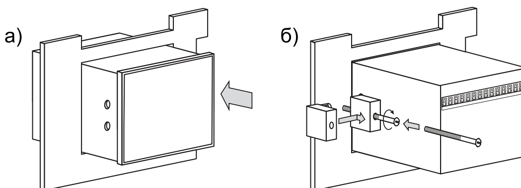
Рисунок 4.4 – Монтаж преобразователя щитового исполнения
