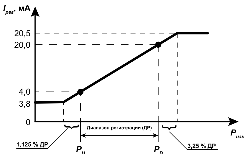
Рисунок 7.3 – Принцип формирования тока регистрации
