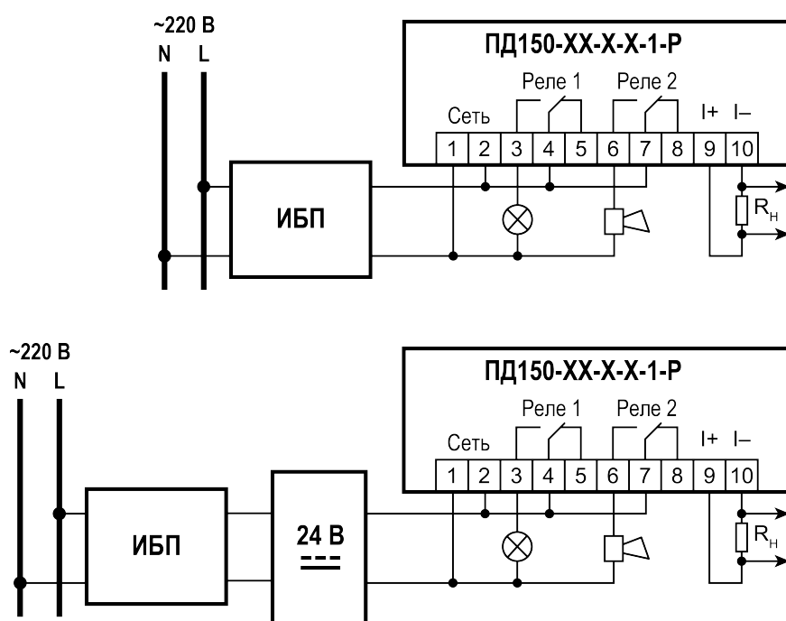
Рисунок 5.6 – Пример схемы подключения преобразователя с аналоговым выходом через ИБП
