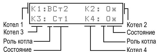
Рисунок 10.13 – Отображение ролей котлов на индикаторе
