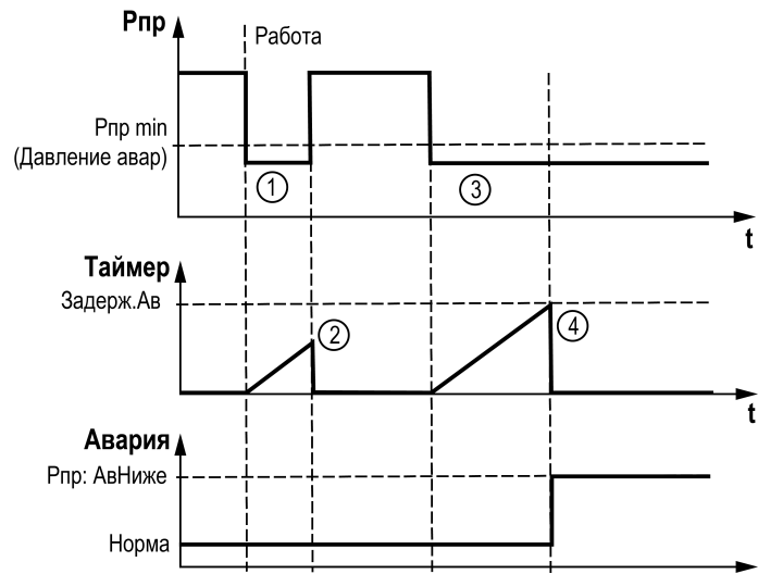
1 — при переходе в режим Работа давление ниже Pпр min , авария не фиксируется, запущен таймер Задерж.Ав ; 2 — давление вернулось в норму до окончания отсчета, таймер сброшен, авария не фиксируется; 3 — давление снова ниже Pпр min , таймер запущен повторно; 4 — условие сохранялось все время отсчета, по окончании Задерж.Ав фиксируется авария Рпр: АвНизже .
