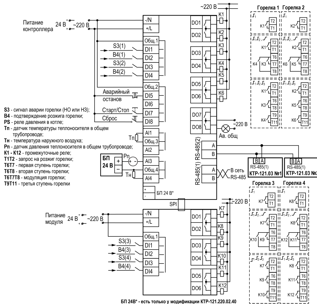
Рисунок 7.4 – Схема подключения КТР-121.02.40 и ПРМ-1 для управления котельной с четырьмя котлами и ГВС
