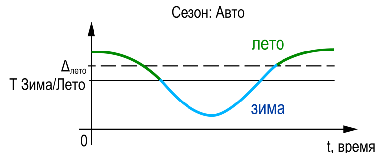
Рисунок 10.4 – Определение сезона
