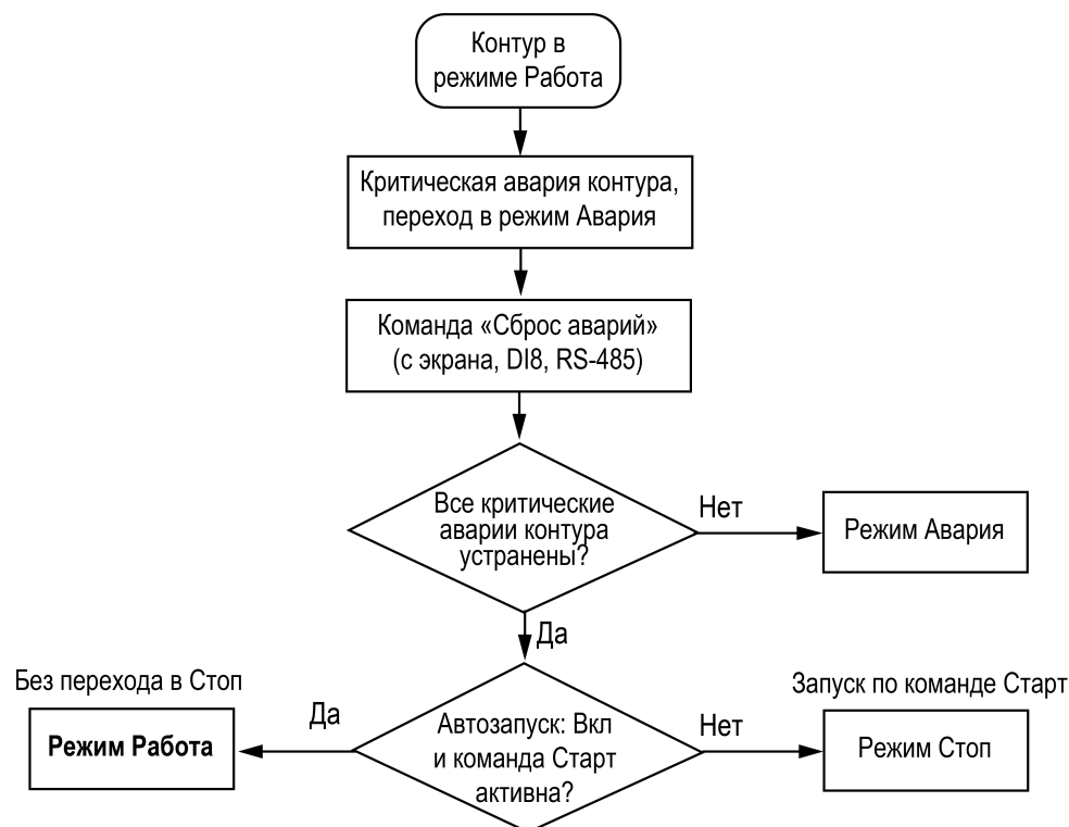
Рисунок 11.1 – Автозапуск контура после критической аварии
