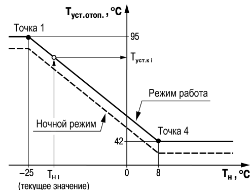
Рисунок 10.3 – График зависимости температуры сдвига от наружной температуры
