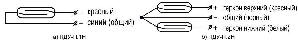
Рисунок 4 – Схемы внутренних соединений проводов
