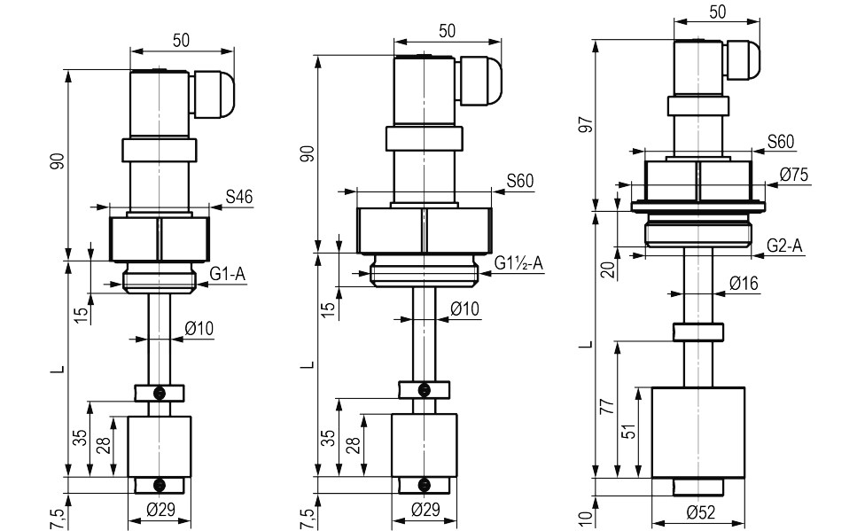
Рисунок 2 – Габаритные и присоединительные размеры одноуровневых ПДУ-П с разъёмом DIN 43650 А (наружный монтаж)
