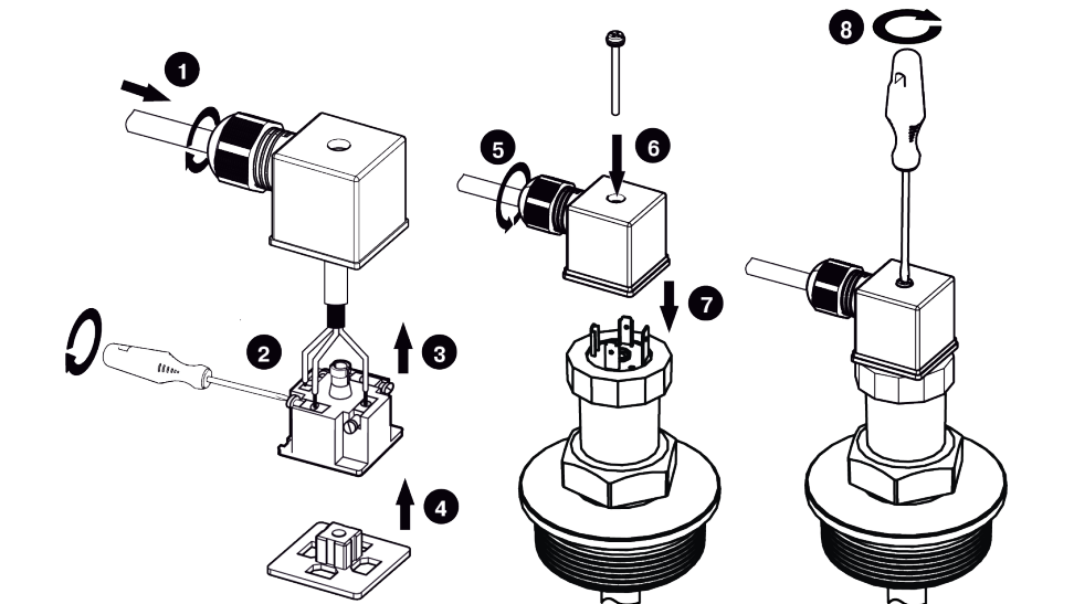
Рисунок 6 – Монтаж проводов датчика с разъемом
