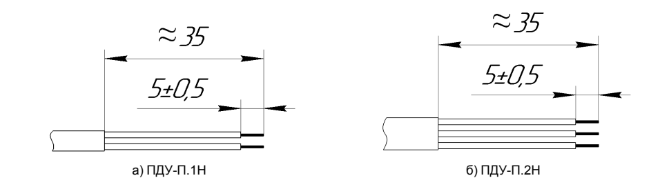
Рисунок 5 – Подготовка кабеля
