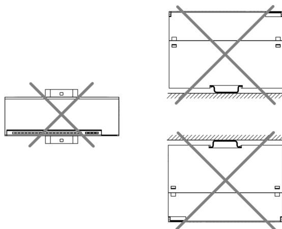
Рисунок 4.2 – Неверный монтаж
