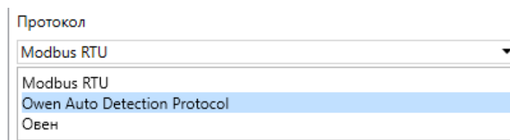
Рисунок 7.3 – Выбор протокола
