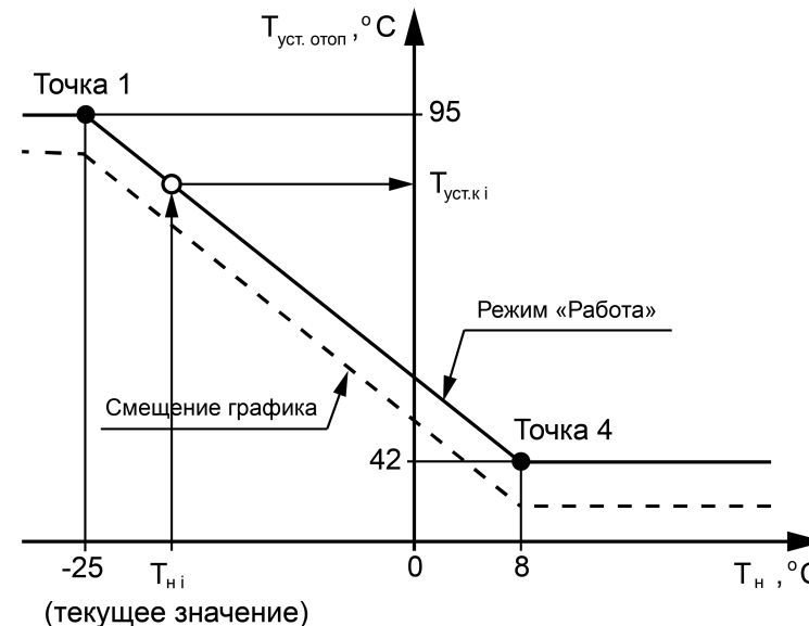
Рисунок 9.7 – Отопительный график
