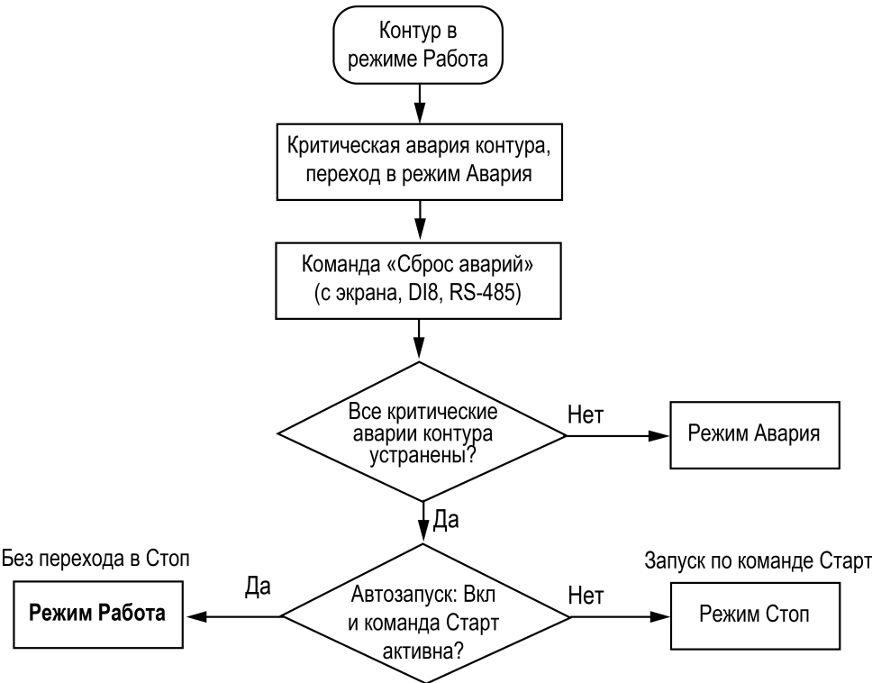
Рисунок 9.11 – Автозапуск контура после критической аварии
