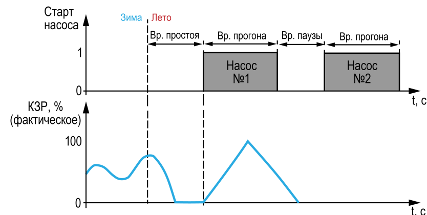
Рисунок 9.9 – Прогон при сезоне «Лето»
