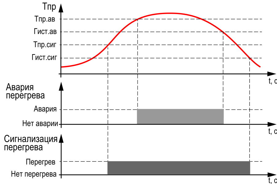
Рисунок 9.10 – Принцип определения и сброса аварии и сигнализации перегрева
