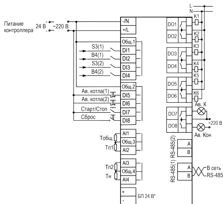
Рисунок 6.4 – Схема подключения КТР–121.02.23 для управления котельной с двумя котлами и контурами ГВС
