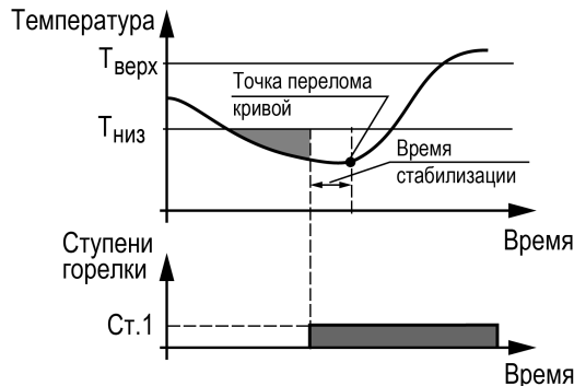
Рисунок 10.11 – Принцип определения Вр.Стаб
