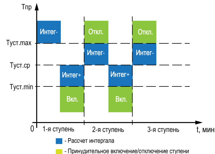
Рисунок 10.5 – Диапазоны расчета интеграла на подключение и отключение для каждой ступени
