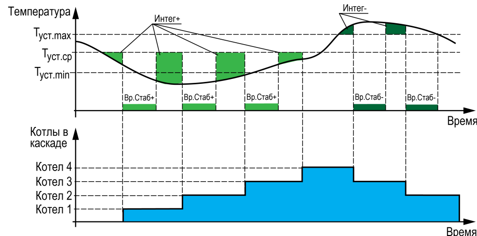
Рисунок 10.9 – Регулирование температуры
