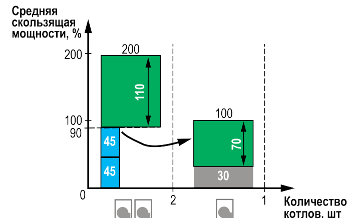
Рисунок 10.10 – Изменение мощности каскада
