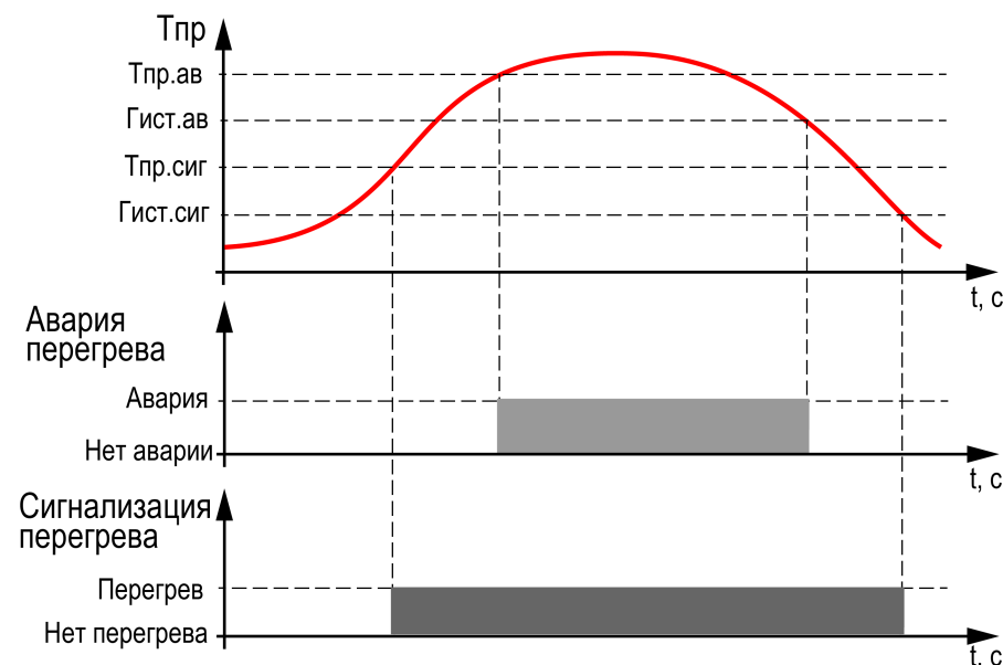
Рисунок 10.13 – Принцип определения и сброса аварии и сигнализации перегрева
