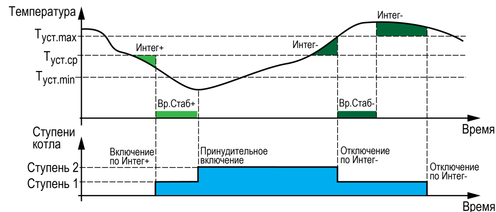
Рисунок 10.4 – Регулирование температуры
