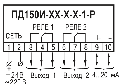
Рисунок 5.2 – Назначение контактов клеммника преобразователя с аналоговым выходом
