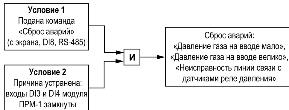
Рисунок 11.1 – Сброс аварий по давлению газа
