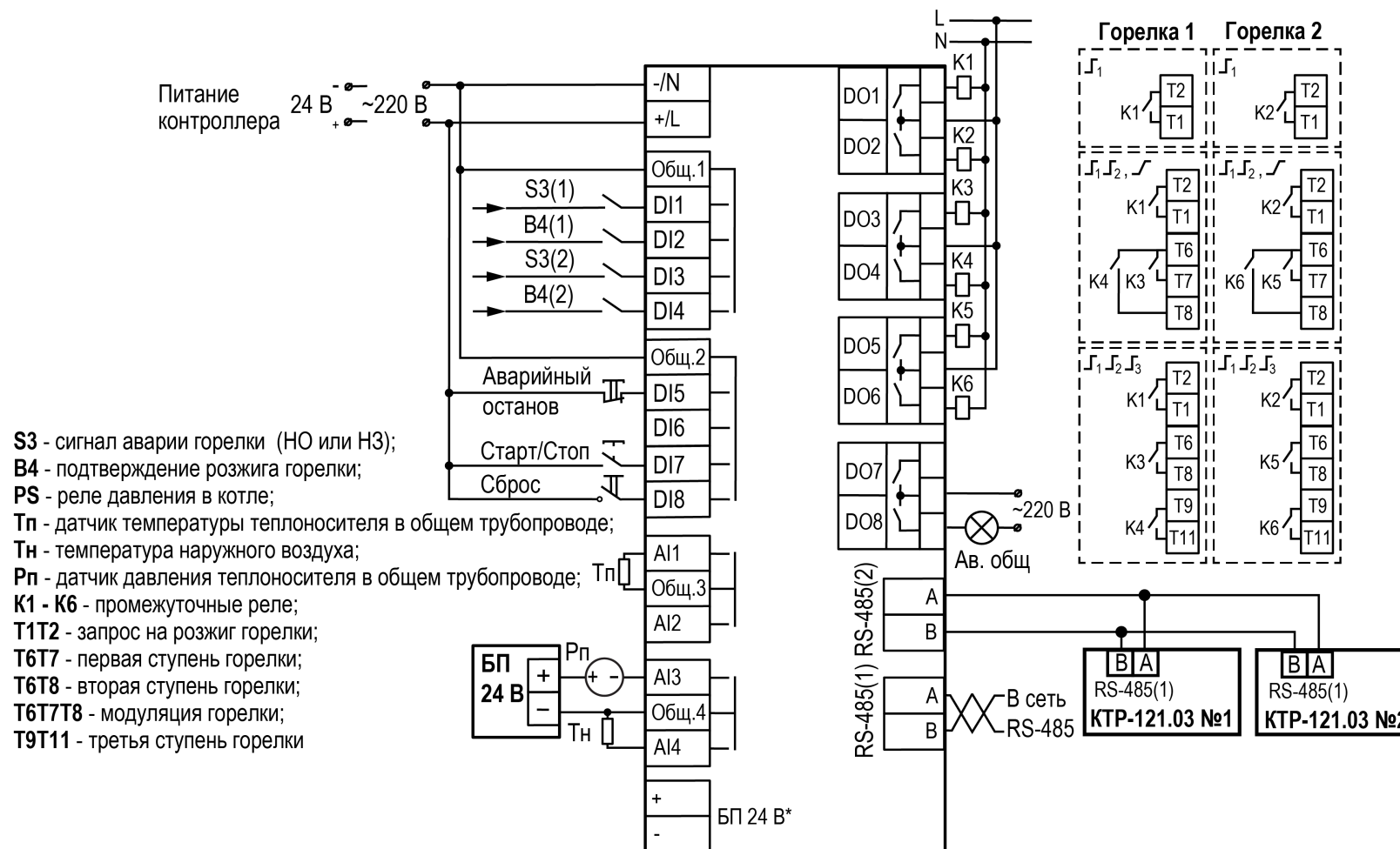
Рисунок 7.4 – Схема подключения KTP-121.02.20 для управления котельной с двумя котлами и контурами ГВС
