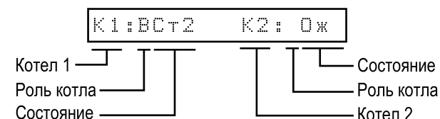
Рисунок 10.13 – Отображение ролей котлов на индикаторе
