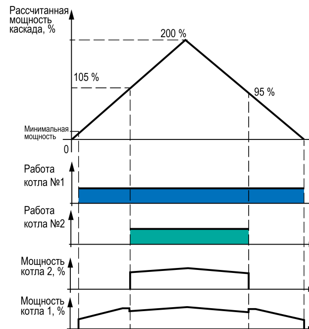
Рисунок 10.7 – Работа каскада котлов с модулируемыми горелками
