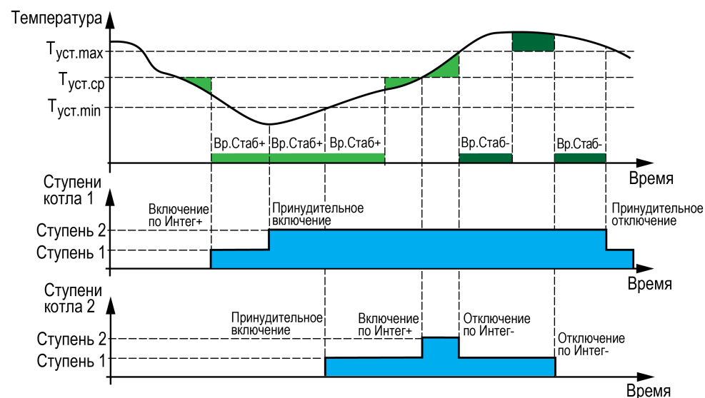
Рисунок 10.2 – Регулирование температуры
