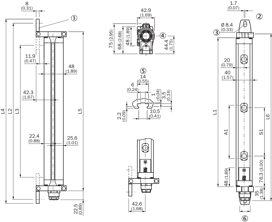
Размеры, мм
