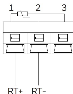
NTC10K/NTC20K/PT1000 两线
